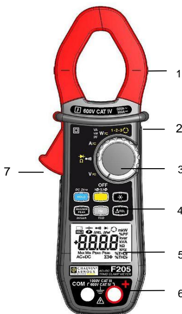
Figur 1: F205 Tångmultimeter
