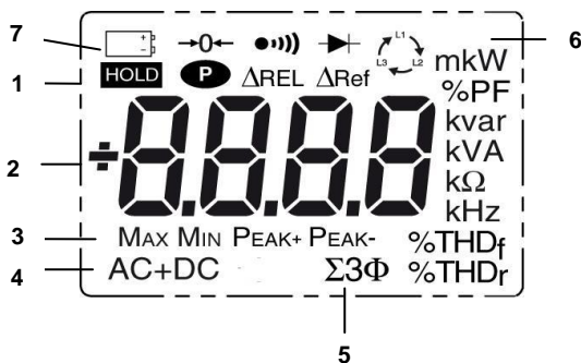
Figur 4: Displayenheten
